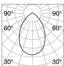
CRI≥80 14W 70° 1600lm 3000K
