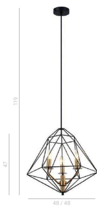
PEN-6369-3-BKBR ⚡ E14 3x40W
