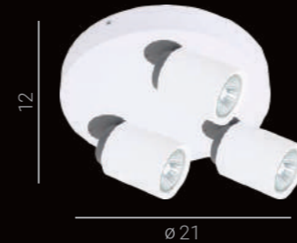
FH31313B GU10 3x35W
