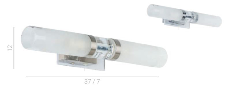
● MB030101-2SN ● MB030101-2C E14 2x40W IP44
