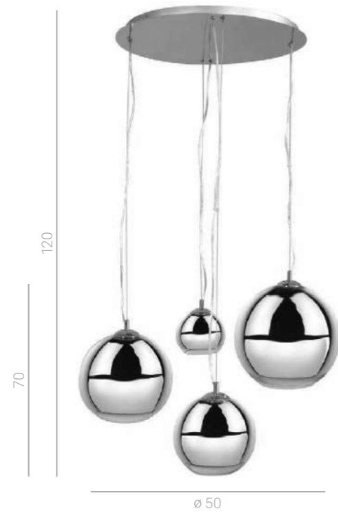
MA04914C-004 ⚡ E27 4x40W
