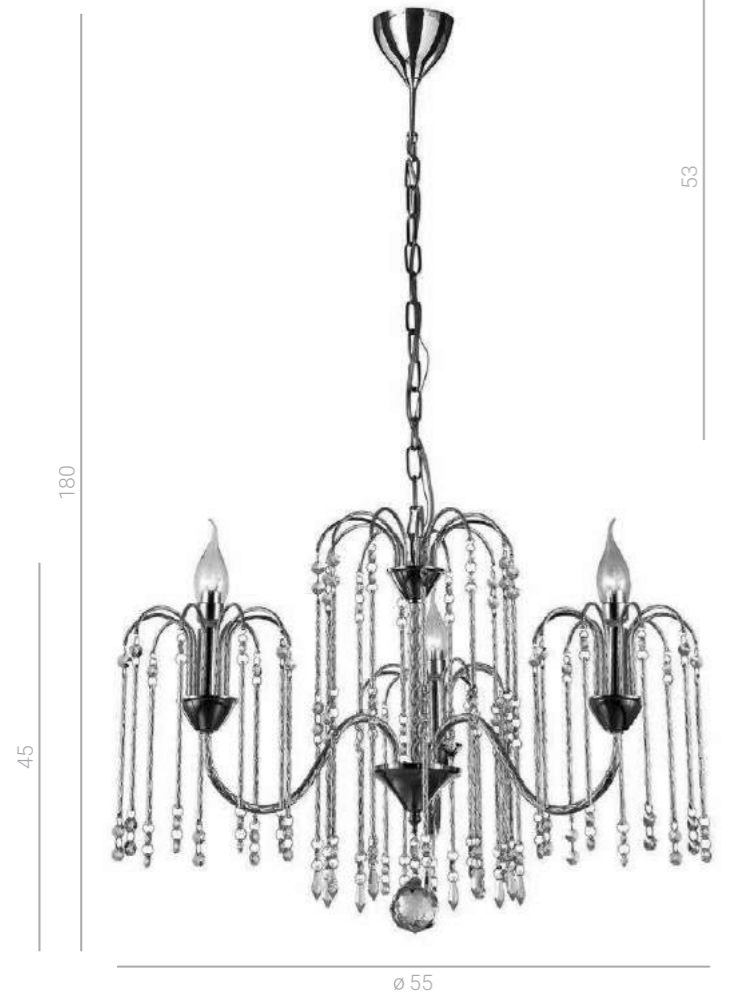
P0354-03B-F4QL E14 3x40W
