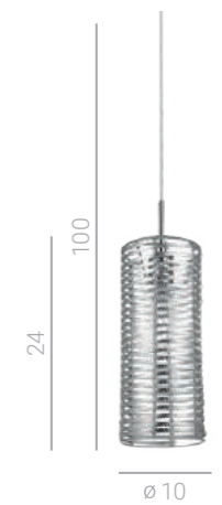
MDM2131/1S SL Ø E14 1x40W
