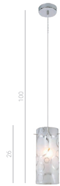
MBM1674/1 W ⚡ E27 1x60W
