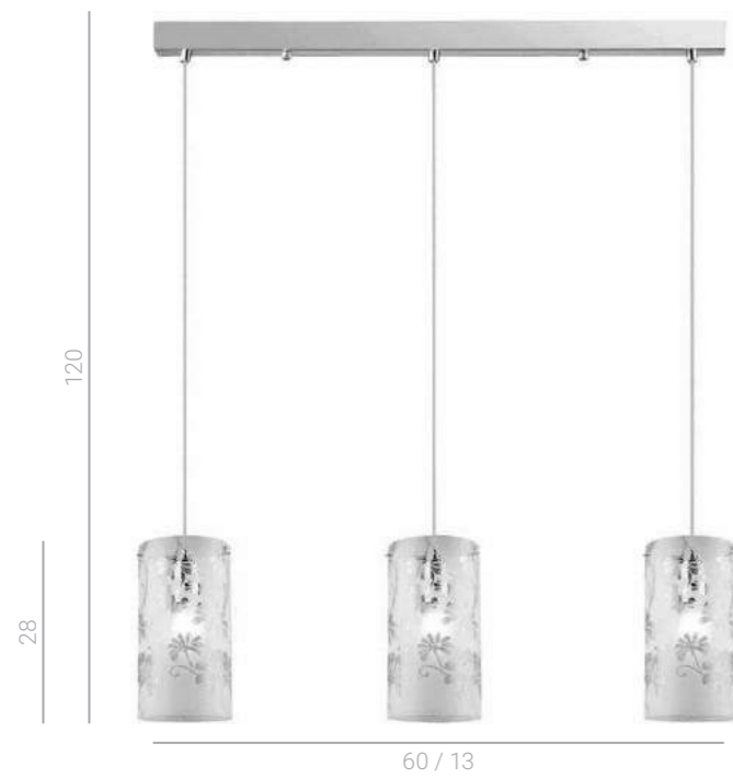
MDM1673-3 ⚡ E27 3x60W
