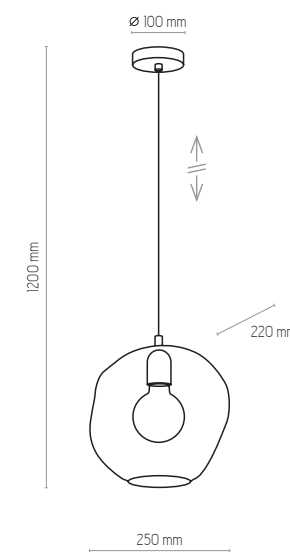
3369 | SOL | 1x E27, max 60W | KL 7781
