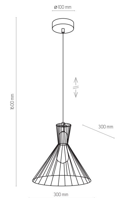
3350 | SAHARA | 1 x E27, max 60W
